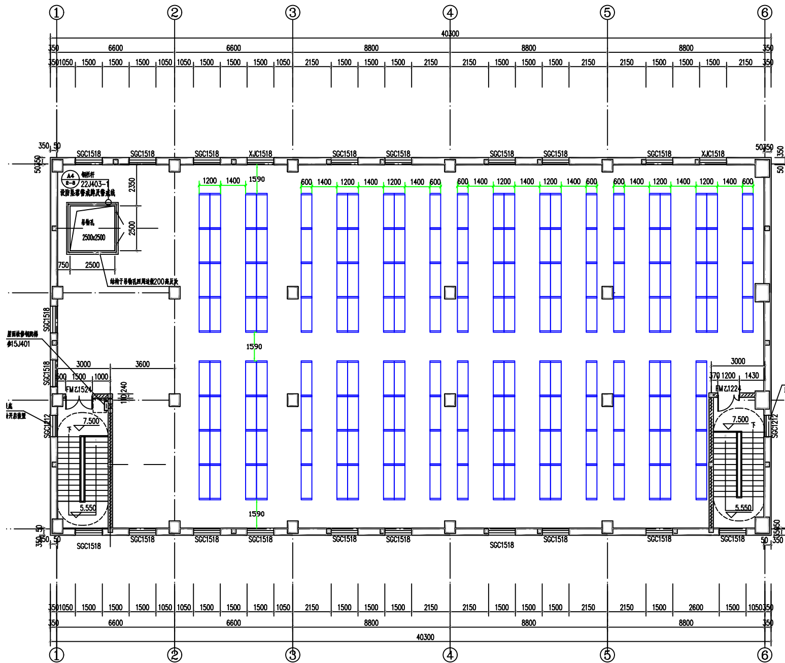
7.500米层平面图
